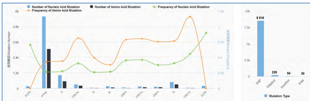
Рис. 10. Число, скорость и типы мутаций коронавируса SARS-CoV-2. По состоянию на 27.05.2020.
