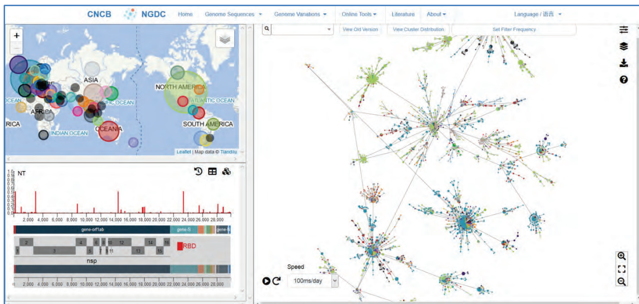
Рис. 8. Интерактивная карта генотипирования коронавируса SARS-CoV-2. Галотипы в мире. По состоянию на 13.05.2020.
