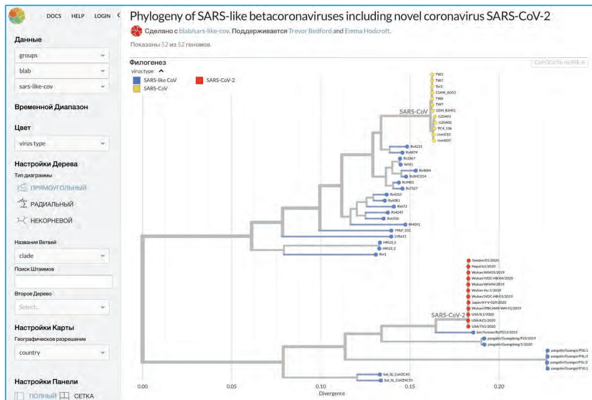
Рис. 6. Филогенетическая ситуация nCoV у SARS-связанных бета-коронавирусов.
